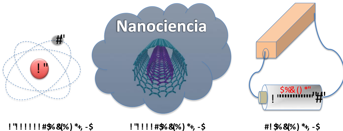
Figura 2 Nanociencia, estudio y manipulación de objetos con dimensiones mucho mayores que las de un átomo pero mucho más pequeñas que las de un objeto macroscópico.
